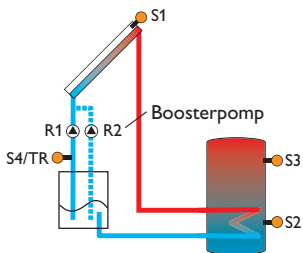
Voorbeeldschema voor een drainback-installatie (R2 = boosterpomp)
